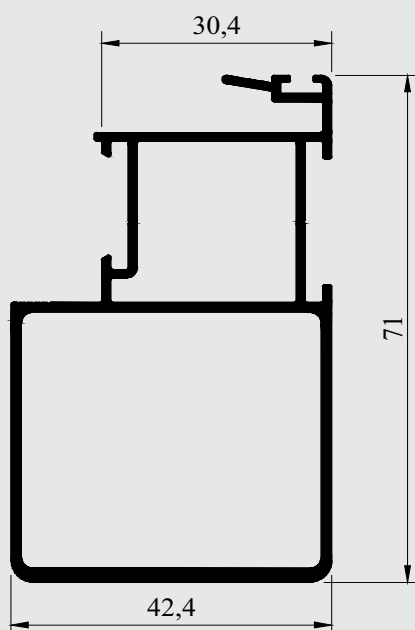
Montante bitubular com baguete
