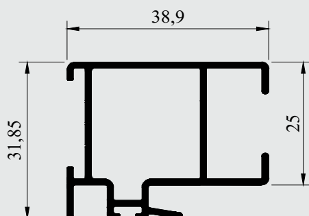
Montante com engate interno e externo sem baguete
