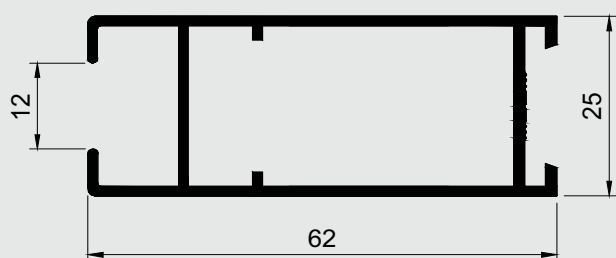
Montante da folha sem baguete
