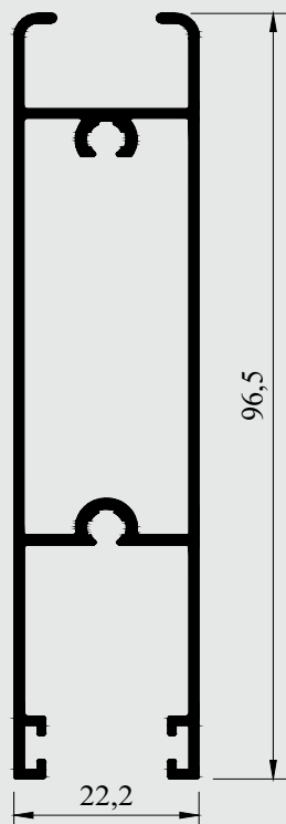
Travessa inferior sem baguete
