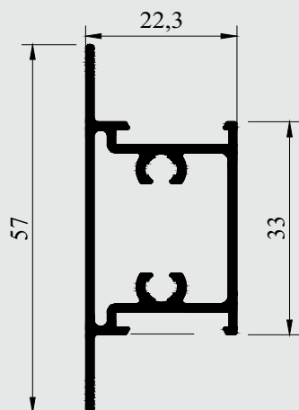
Montante da folha sem baguete
