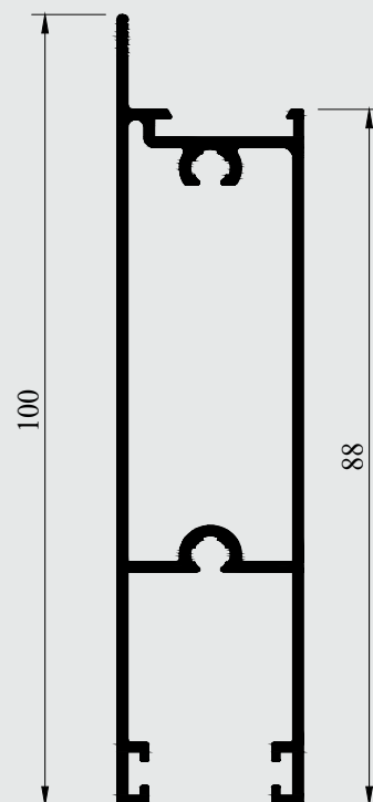
Travessa inferior com baguete
