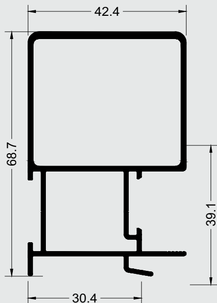
Montante bitubular com baguete
