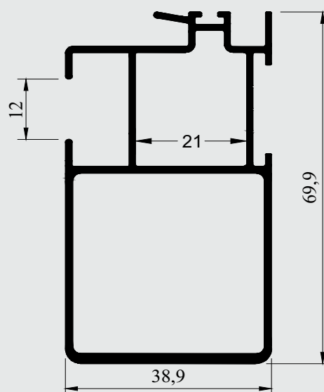
Montante com engate interno e externo sem baguete
