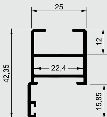
Montante da folha sem baguete
