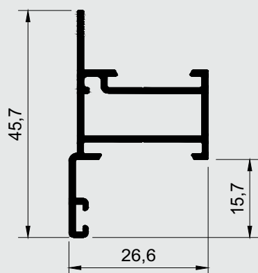
Montante da folha com baguete
