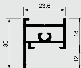
Montante superior 90° com baguete
