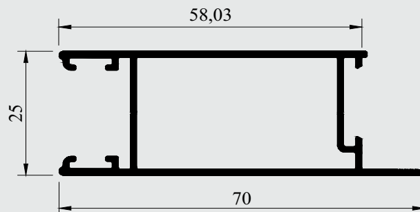
Montante Vertical pV fechadur
